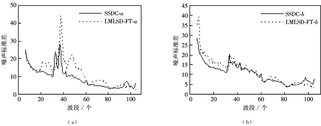
图 9 利用基于高斯波形提取的 LMLSD 对图 1 中 AVIRIS 辐射图像进行噪声评估的结果 Fig 9 Estimations of the noise for AVIRIS radiance images shown in Figure 1 via LMLSD based on Gaussian distribution pick-up
