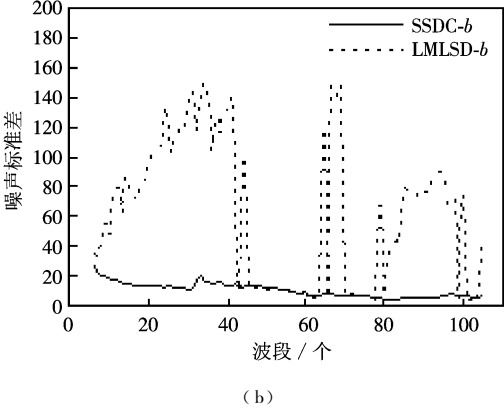
图 3 采用 LMLSD 和 SSDC 对 AVIRIS 辐射图像进行噪声评估
